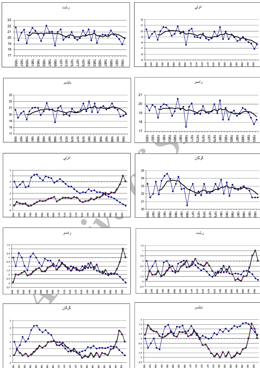
شکل ۱- تغییرات آماره های U و U' و میانگین متحرک ۵ ساله دمای متوسط حداکثر فصلی در ایستگاه های مورد مطالعه
