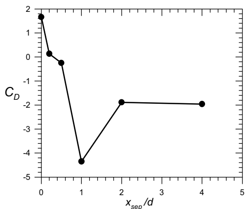
شکل ۹- ضریب نیروی مقاوم روی سرچنگی در فواصل مختلف سر و بدنه
