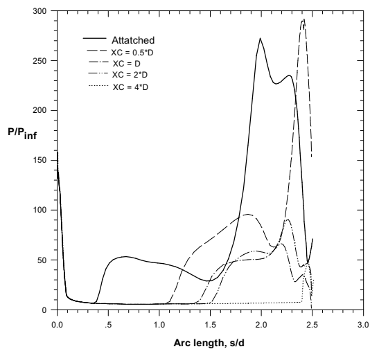
شکل ۸- توزیع فشار بر روی سطح سرچنگی برای حالت متصل و فواصل مختلف سر و بدنه
