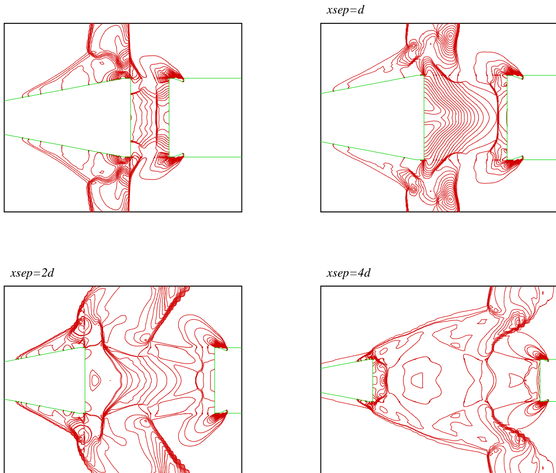
شکل ۶- خطوط همتراز فشار در فواصل مختلف سر و بدنه
