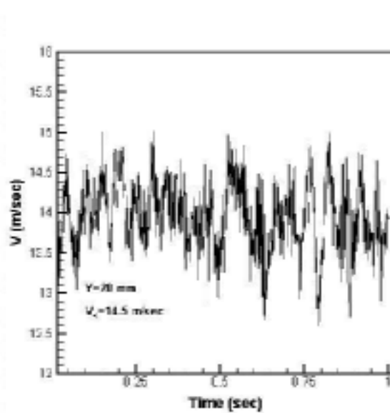
شکل ۱۳-الف- تغییرات سرعت با زمان در داخل هسته گردابه
