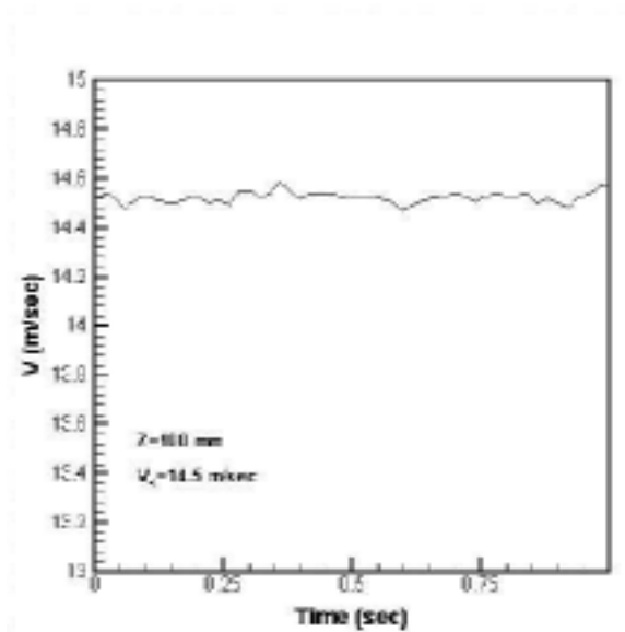
شکل ۱۳-ب- تغییرات سرعت با زمان در خارج هسته گردابه
