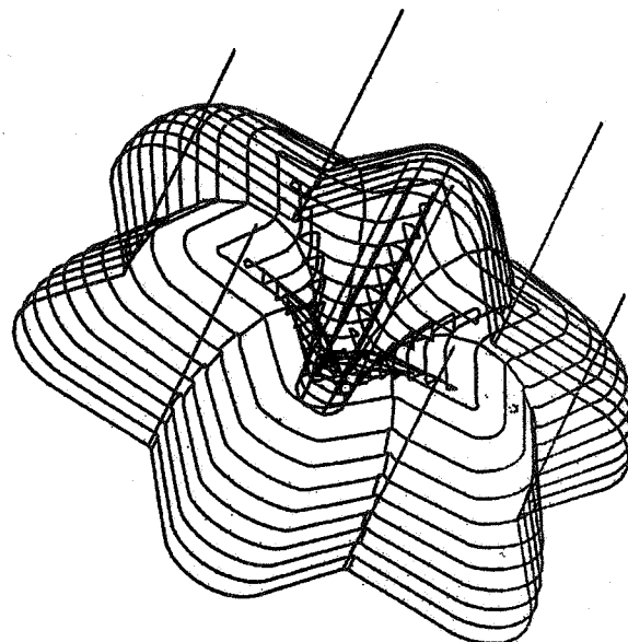
شکل ۱۴- نمونه‌ای از یک رویه پیچیده با استفاده از معادله Z = f(X, Y) و مسیرهای ماشینکاری آن
