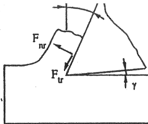
شکل ۱- نیروهای اصلی ایجاد شده در ماشینکاری
