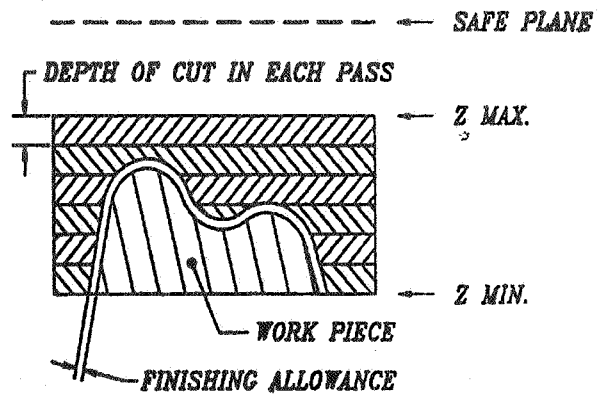
شکل ۱۳ - بعضی از پارامترهای تراش
