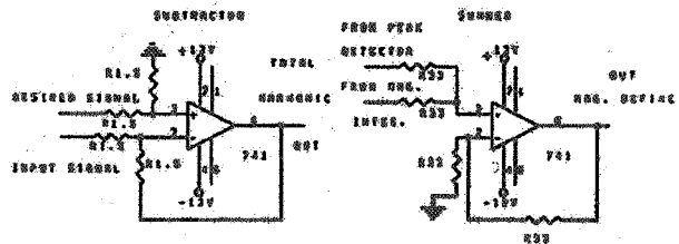
شکل ۱۷- شماتیک مدارهای جمع کننده و تفریق کننده
