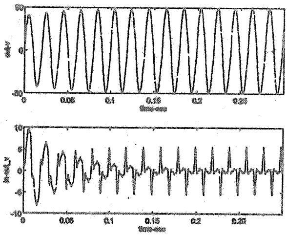
شکل ۷- شکل موج‌های خروجی (تخمین مؤلفه اصلی ورودی) و اختلاف خروجی با ورودی در شرایطی که فرکانس مؤلفه اصلی ورودی ۵۰/۵ هرتز باشد ولی فرکانس VCO در شبیه‌سازی ۵۰ هرتز باشد و با روش دیگری خارج الگوریتم وقتی نیز فرکانس دنبال نشود.
