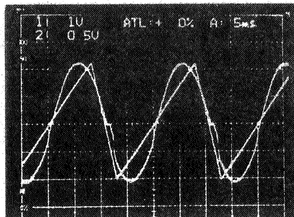
شکل ۲۱- استخراج مؤلفه اصلی سیگنال دندانان اراهی با فرکانس ۵۰ هرتز
