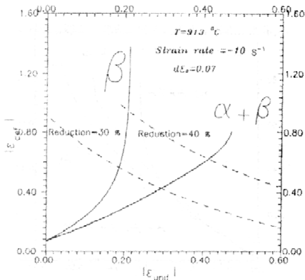
شکل ۷- کرنش در ناحیه معیوب بر حسب کرنش در ناحیه غیر معیوب برای آلیاژ Ti-6242 Si با دو ساختار میکروسکوپی مختلف در شرایط نشان داده شده
