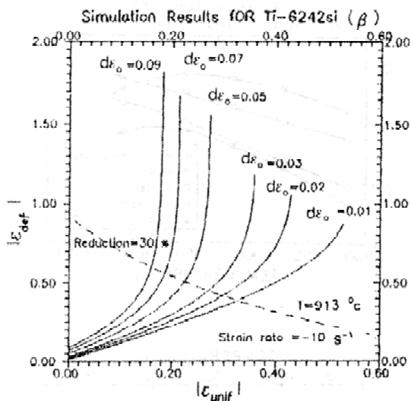
شکل ۹- کرنش در ناحیه معیوب بر حسب کرنش در ناحیه غیر معیوب برای آلیاژ (β) Ti 6242 Si در T=913°C و \dot{\epsilon}_0 = 10s^{-1} برای d\epsilon_0 های نشان داده شده
