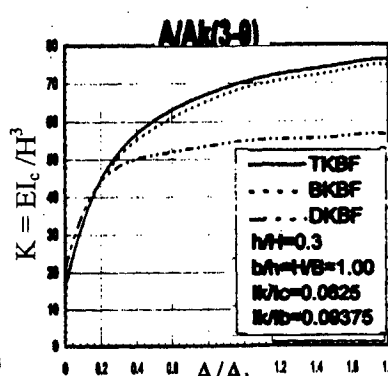
الف- تغییرات A/A_k
