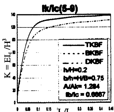
ج- تغییرات I_k/I_c
