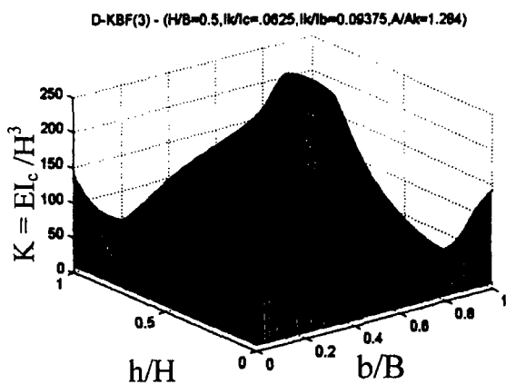
شکل ۵- یک نمونه از سطح سه بعدی سختی و منحنیهای هم سختی سیستمهای DKBF. H/B=0.5 .
