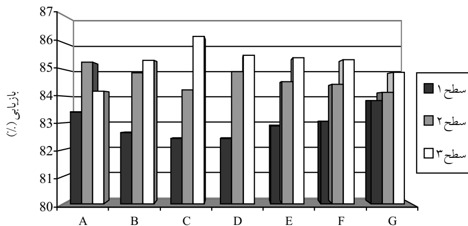
شکل ۱- تأثیر سطوح هفت عامل در بازایی سنگ معدن کالکوسیتی
