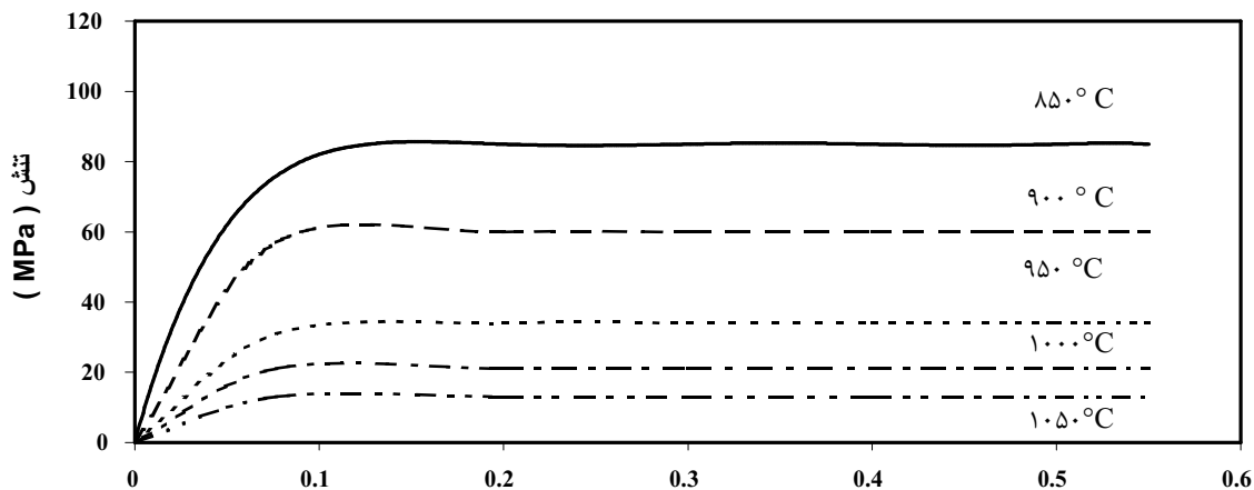
شکل ۷- منحنی تنش کرنش حقیقی در آهنگ کرنش 10^{-2} (1/s)
