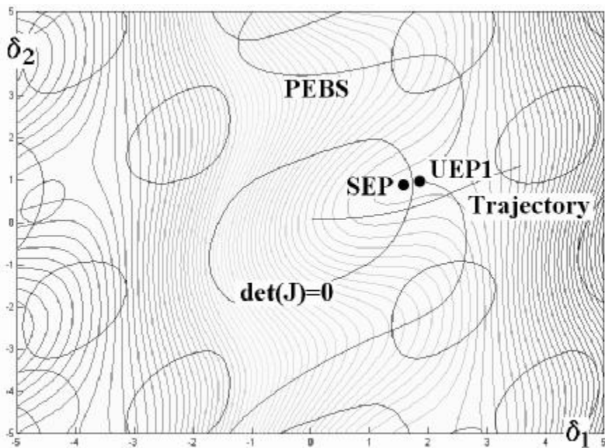
شکل ۴- سیستم تحت فشار در ازای افزایش P_{m1}
