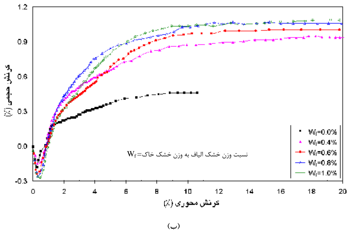
شکل ۵- تغییرات تنش انحرافی (شکل الف) و کرنش حجمی (شکل ب) در آزمایش سه محوری CD ( s'_c = 100 \text{ kPa} ) برای درصدهای وزنی مختلف عناصر تسلیح ( W_f ) و نسبت اضلاع عناصر A_R = 7
