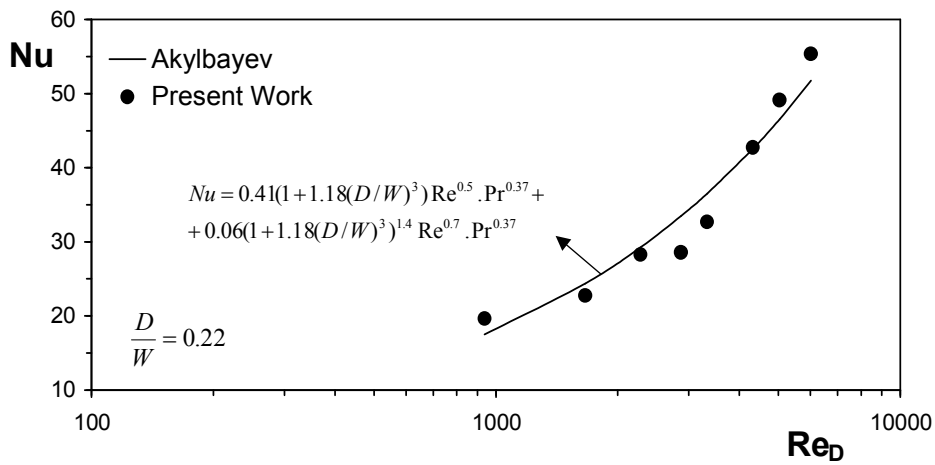
شکل ۵- تغییرات عدد ناسلت یک لوله داخل کانال
