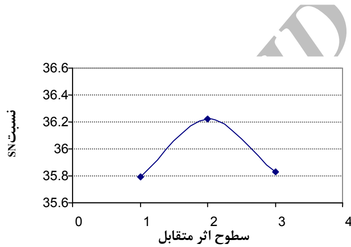
شکل ۱۶- تأثیر اثر متقابل نسبت مایع به جامد و دما، ظاهر شده در ستون نهم آرایه بر نسبت SN
