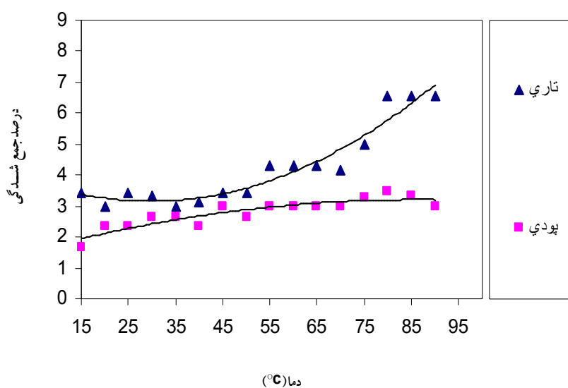
شکل ۵- نمودار تغییرات درصد جمع شدگی نمونه‌های قلیایی شده در دو جهت تاری و بودی برحسب دما در غلظت C=260\text{gr/li} و زمان t=5\text{min}
