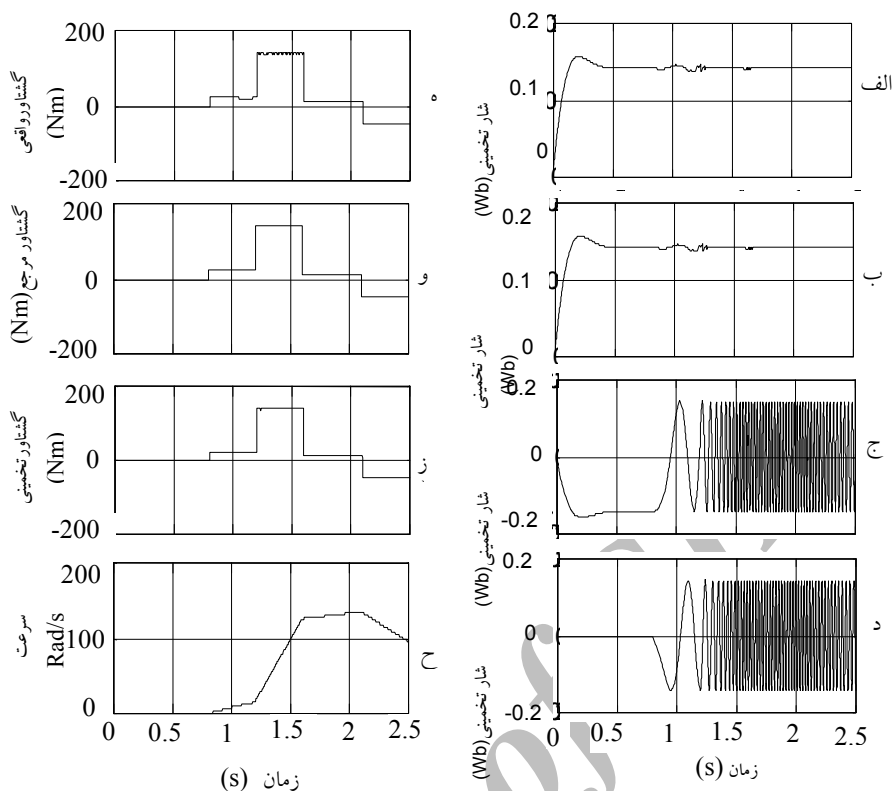
شکل ۹. عملکرد سیستم با استفاده از انگرال گیر پیشنهادی برای حل مشکل dc offset الف- شار واقعی ب- شار تخمینی ج- مؤلفه شار تخمینی در محور d د- مؤلفه شار تخمینی در محور q ه- گشتاور واقع و- گشتاور مرجع ز- گشتاور تخمینی ح- سرعت
