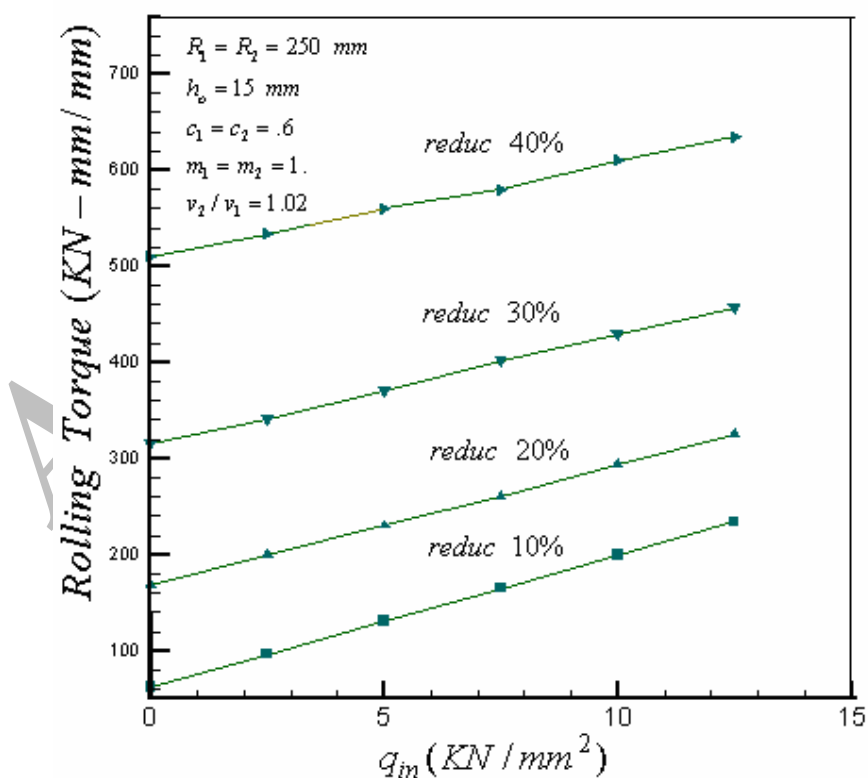
نمودار ۱۰-ب اثر کشش از پشت بر گشتاور لازم برای نورد
