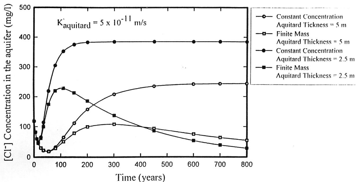
شکل ۶ - تغییرات غلظت یون کلر (Cl) در سفره آبدار نسبت به زمان در مدفن زباله غیرمهندسی (گزینه اول). (۱) تاثیر غلظت ثابت نسبت به غلظت یا جرم محدود در کف مدفن، (۲) تاثیر ضخامت لایه زمین طبیعی
