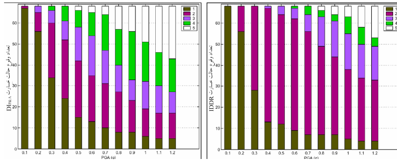
شکل ۲۱- تعداد وقوع حالات خسارت وابسته به توابع IDDR و DI_{P\&A} در سطوح مختلف شتاب حداکثر زمین
