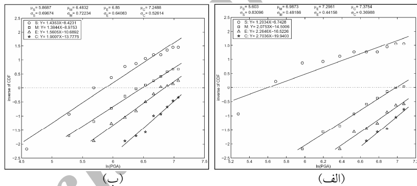
شکل ۲۳- ترسیم تعداد وقوع حالات خسارت وابسته بر توابع IDDR و DI_{P\&A} در سطوح مختلف شتاب حداکثر روی کاغذ احتمال لوگ-نرمال
