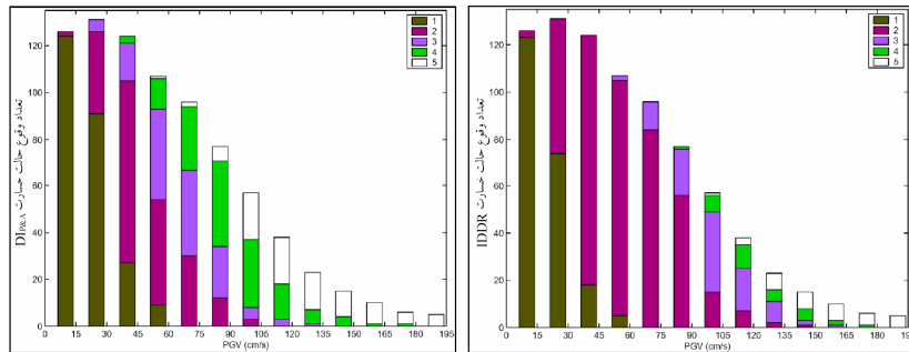
شکل ۲۲- تعداد وقوع حالات خسارت وابسته به توابع IDDR و DI_{P\&A} در سطوح مختلف سرعت حداکثر زمین
