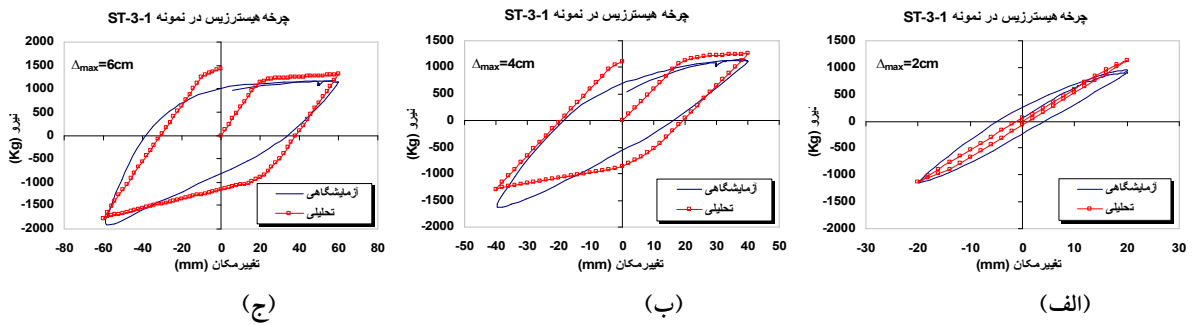
شکل ۱۰- مقایسه رفتار هیسترتیک در مطالعات آزمایشگاهی و تحلیلی در نمونه ST-3-1 در یک چرخه کامل بارگذاری الف) دامنه تغییر مکان ۲ سانتیمتر ، ب) دامنه تغییر مکان ۴ سانتیمتر، ج) دامنه تغییر مکان ۶ سانتیمتر
