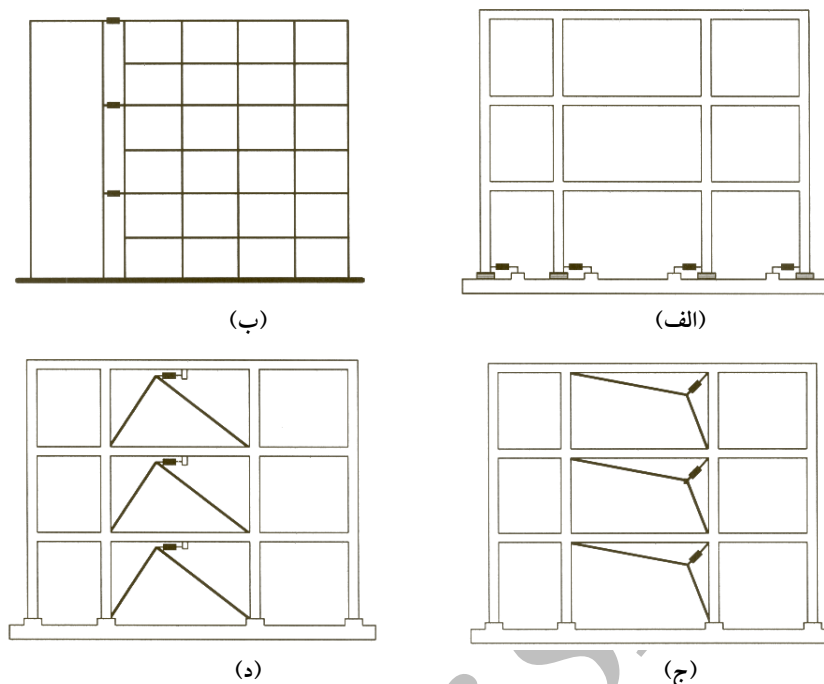
شکل ۲۵- کاربرد میراگر فلزی آکاردئونی در مقاوم سازی لرزه‌ای قابها و موقعیت قرارگیری آنها الف) استفاده در جداسازی لرزه‌ای، ب) استفاده در کنترل تغییر مکانهای مطلق طبقات، ج) استفاده در بادبندهای با مکانیسم تغییر شکل بزرگ، د) استفاده در بادبندهای شورن و کنترل تغییر مکان نسبی طبقات
