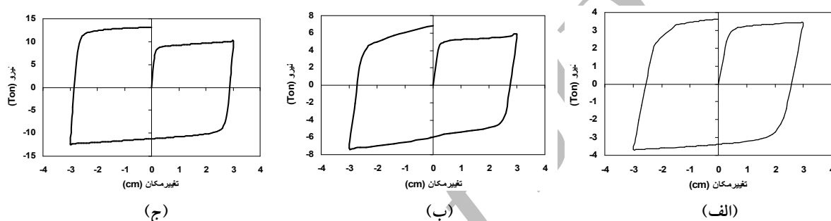
شکل ۱۴- رفتار هیسترتیک در تحلیل اجزای محدود لوله‌های جدار نازک آکاردئونی
