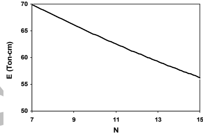
شکل ۲۱- تأثیر تعداد پلیسه‌ها بر اتلاف انرژی لوله آکاردئونی با جداره دایره‌ای شکل
