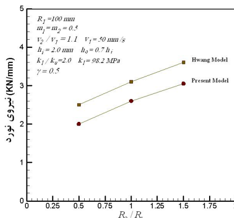
شکل ۲۰- مقایسه برآورد نیروی نورد در مدل حاضر
