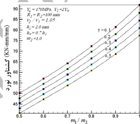
شکل ۱۰- تغییرات گشتاور نورد بر اساس نسبتهای مختلفی از ضرایب اصطکاک دو غلتک و نسبت ضخامتهای مختلفی از دو لایه
