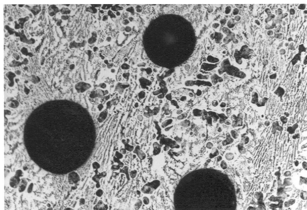
شکل ۴- حفرات گازی در نمونه Fe-10%Ti-3%C ریخته‌گری شده در قالب سرامیکی به روش گریز از مرکز، ساختار زمینه؛ پرلیت، محلول اچ: نایتال ۲ درصد، قالب سرامیکی
