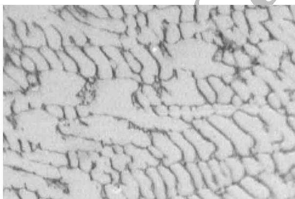
شکل ۸- نمونه عملیات حرارتی شده، دانه‌های فریت در سطح نمونه Fe-10% Ti-3% C، محلول اچ نایتال ۲ درصد
