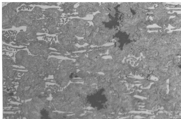
شکل ۶- تشکیل گرافیت برفکی شکل در نمونه آنیل شده Fe-10% Ti-3% C : ساختار زمینه پرلیت، شرایط عملیات حرارتی: گرم کردن نمونه تا ۹۵۰ °C به مدت ۱ ساعت و سرمایش در هوا، ابعاد نمونه: نمونه‌های استوانه‌ای به قطر ۱/۵ و طول ۵ سانتی متر
