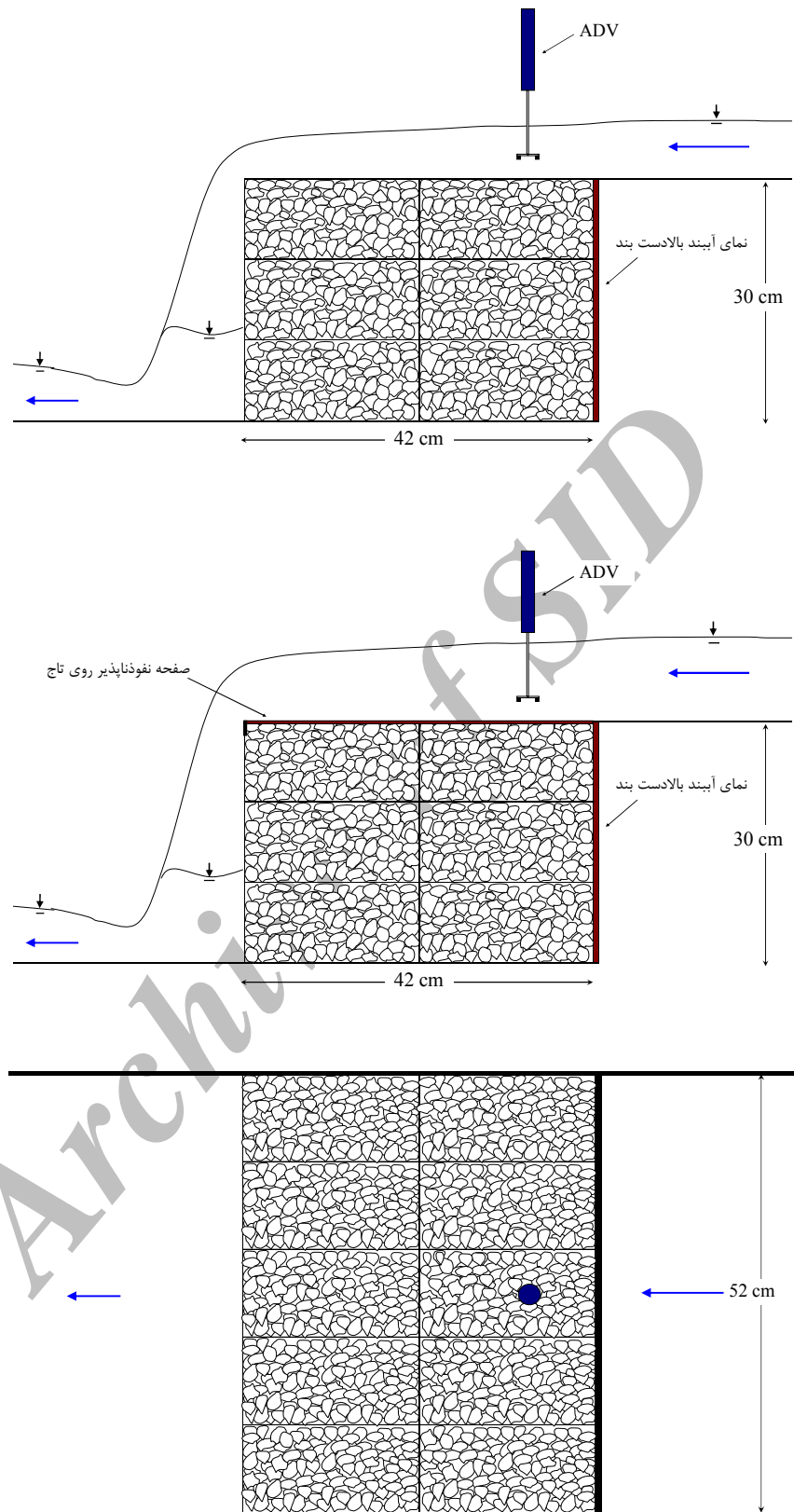
شکل ۴ - شکلهای به ترتیب بالا مقطع طولی بند با تاج نفوذپذیر، وسط مقطع طولی بند با تاج نفوذناپذیر و پایین پلان بند با تاج نفوذپذیر
