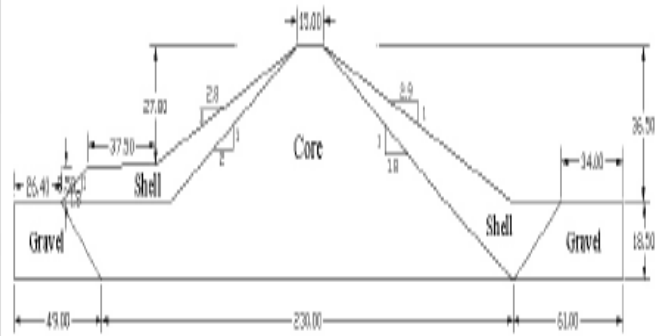
شکل ۱۴ - مشخصات مقطع عرضی سد "لانگولی" شکل ۱۵ - ناحیه بندی در مقطع سد "لانگولی" در نرم افزار "فلک"
