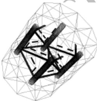
شکل ۸ - سازه دریایی مثال (۲) و محیط اطراف آن پس از شبکه بندی
