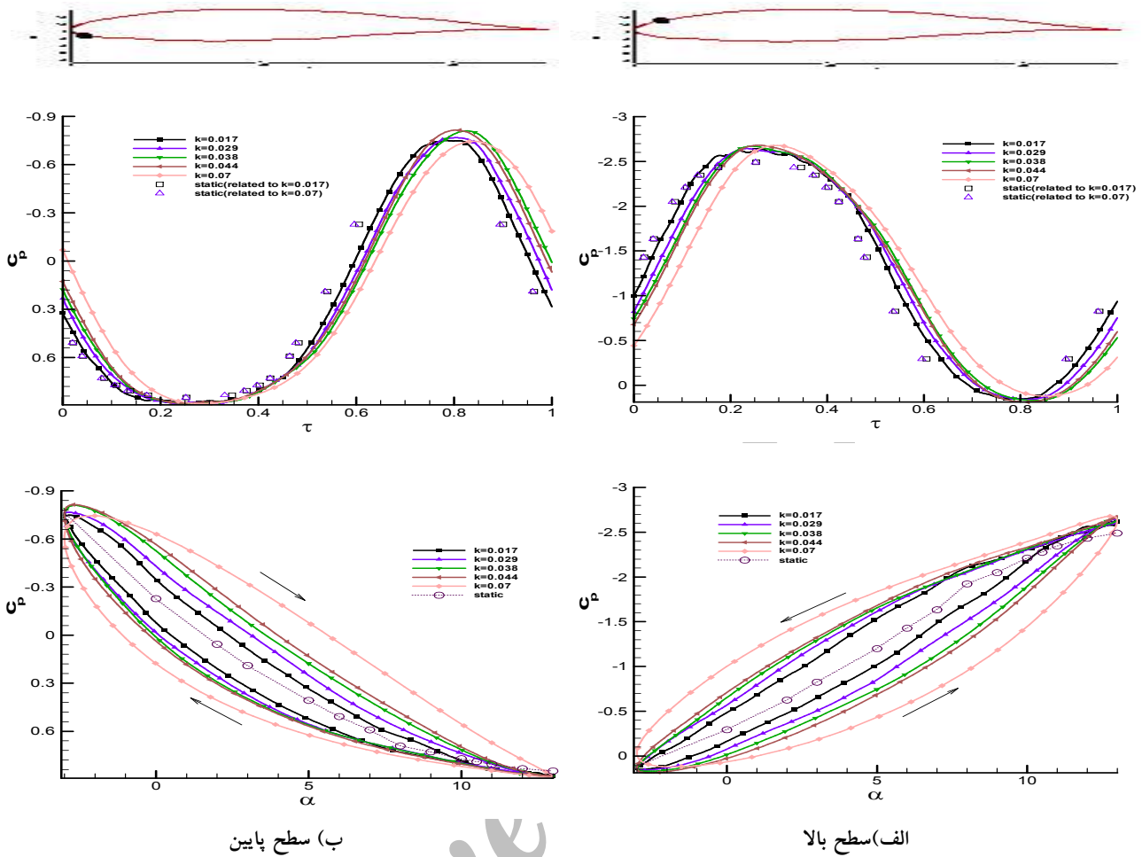
شکل ۱۰-۱ - تاثیر افزایش k در تغییر فشار استاتیکی، \alpha = 5 + 8 \sin(\omega t) & Re = 0.63 \times 10^6 , x/c = 0.05
