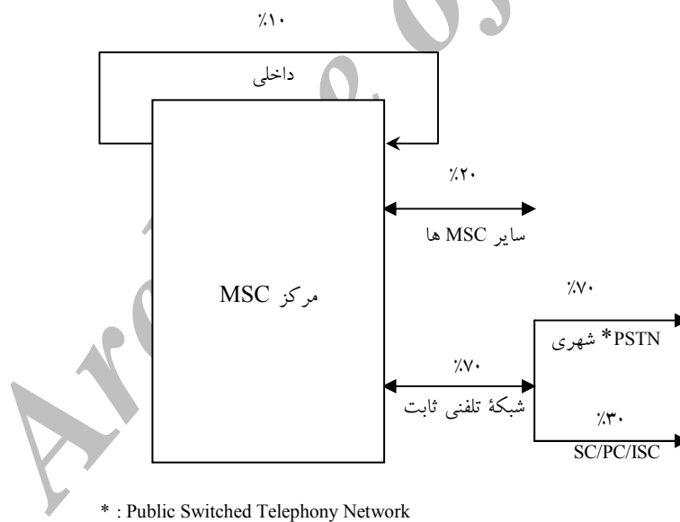
شکل ۴- مدل توزیع ترافیک در MSC
