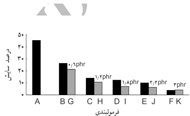
شکل ۶- اثر بررسی اثر فرمولبندی و وجود TAC بر مقاومت سایشی آمیزه: (■) بدون TAC (□) با TAC.
