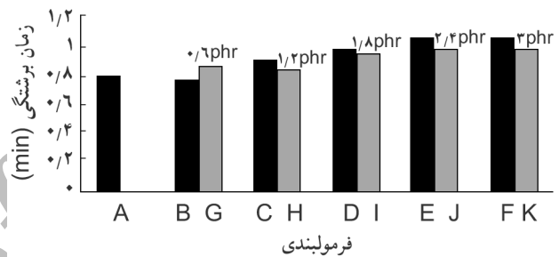
شکل ۲- اثر فرمولبندی و استفاده از TAC بر زمان برستگی آمیزه (مدت زمان لازم برای رسیدن به ۵ درصد پخت کامل): (■) بدون TAC (□) با TAC.
