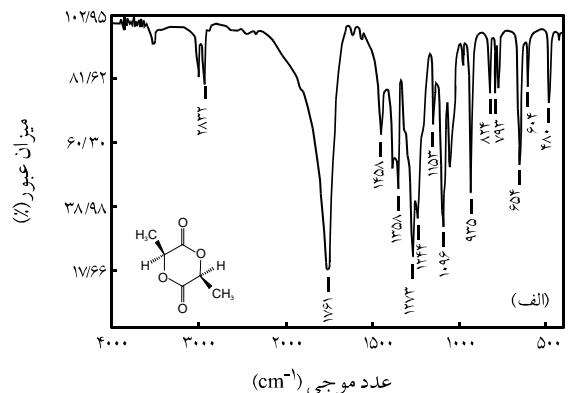
شکل ۱- طیفهای FTIR: (الف) مونومر L-لاکتید و (ب) پلی (L-لاکتید).
