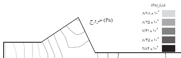
شکل ۴ - توزیع نمودارهای هم اندازه فشار در حیدیه آسترودر آزمایشگاهی ( T = 100^\circ\text{C} و N = 10 rpm).
