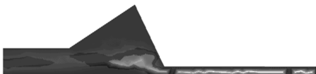
شکل ۶ - توزیع نمودارهای هم اندازه سرعت در آسترودر آزمایشگاهی ( T = 100^\circ\text{C} و N = 40 rpm).
