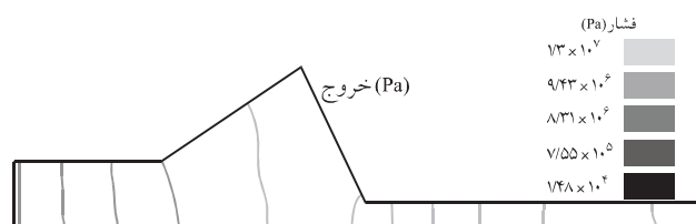
شکل ۵ - توزیع نمودارهای هم اندازه فشار در حیدیه آسترودر آزمایشگاهی ( T = 100^\circ\text{C} و N = 40 rpm).
