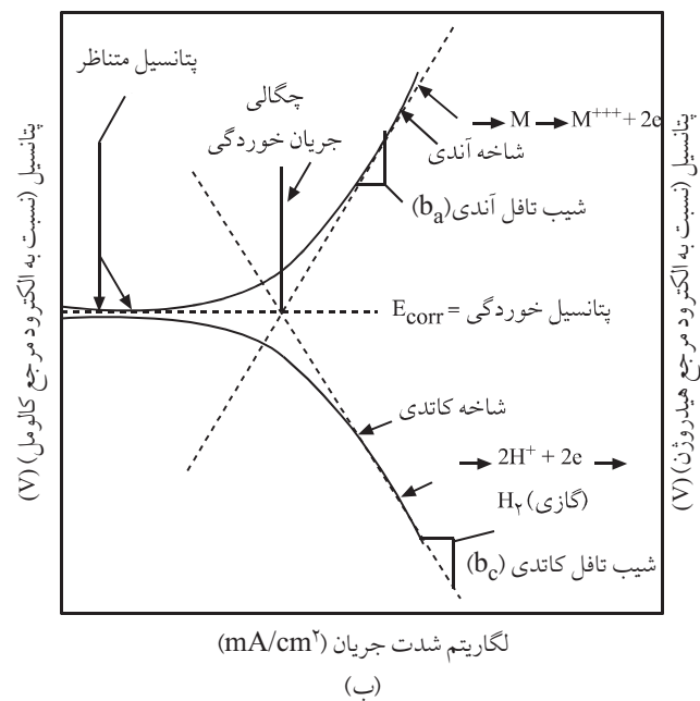
شکل ۷- روش محاسبه مقاومت (الف) و شدت جریان خوردگی (ب) با استفاده از نمودارهای قطبش [۱۰].
