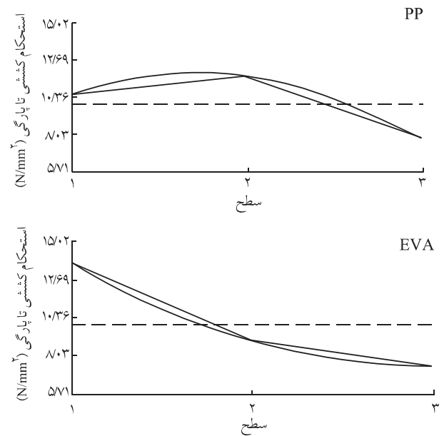
شکل ۳ نمودار تغییرات استحکام کششی تا پارگی بر حسب سطوح.
