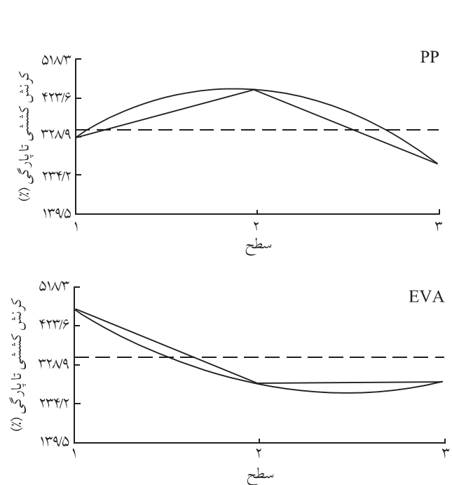
شکل ۴ نمودار تغییرات کرنش کششی تا پارگی بر حسب سطوح.
