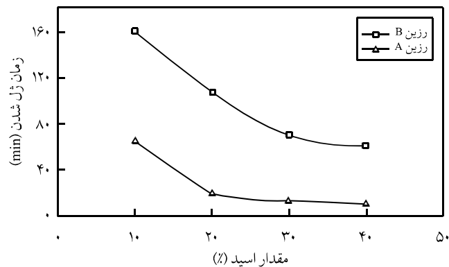
شکل ۳- تغییرات زمان ژل شدن رزین‌های A و B در مقادیر مختلف اسید.
