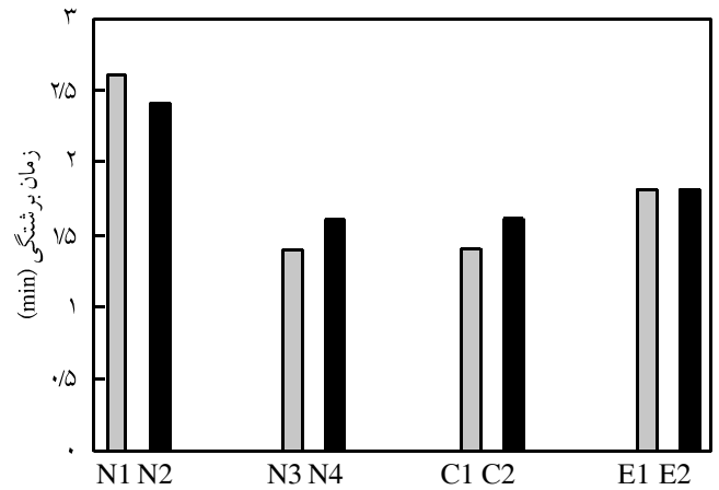
شکل ۴- اثر افزودن الیاف چرم بر زمان برشته‌گی آمیزه‌ها.
