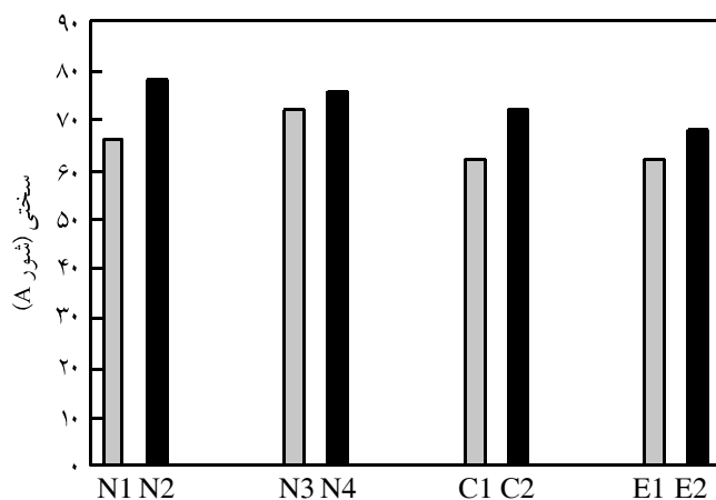
شکل ۷- اثر افزودن الیاف چرم بر سختی آمیزه‌ها.
