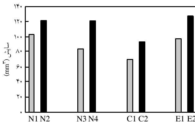
شکل ۹- اثر افزودن الیاف چرم بر مقاومت سایشی آمیزه‌ها.
