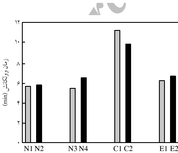
شکل ۳- اثر افزودن الیاف چرم بر زمان پخت آمیزه ها.
