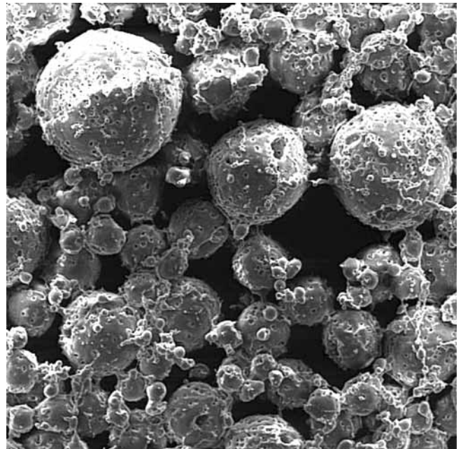
شکل ۳ - شکل شناسی گلوله‌ی مربوط به سامانه پلی (D, L-لاکتیک اسید) - ۴،۱ - دیوکسان - آب با نسبت ۷۵-۸۳-۱۷ در بزرگ‌نمایی ۲۰۰۰X.
