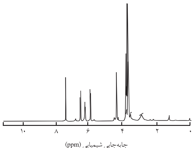
شکل ۲ - طیف 1 H NMR مشتق دی‌آکریلات پلی‌ایتیلن گلیکول ۱۰۰۰.
