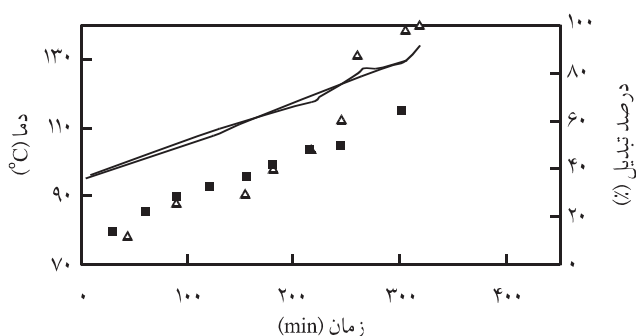
شکل ۵- مقایسه نمودار درصد تبدیل (نقاط گسسته) و برنامه دمایی (نقاط پیوسته) بر حسب زمان برای فرمول بندی حالت دوم مخلوط: (الف) دو آغازگر AIBN و BPO و (ب) دو آغازگر AIBN و TBPB.
