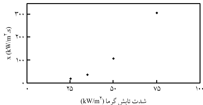
شکل ۱۲ - تغییر x با شدت تابش گرما در اسفنج سخت PUR.
