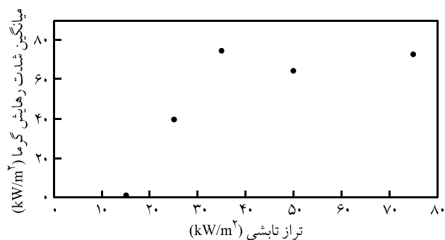
شکل ۷- رابطه Av.RHR اسفنج PUR با شدت تابش گرما.
