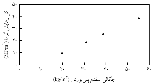
شکل ۱۱ - اثر چگالی اسفنج PUR روی THR.
