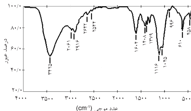
شکل ۳- طیف FTIR کوپلیمر پیوندی CGD (جدول ۱).
