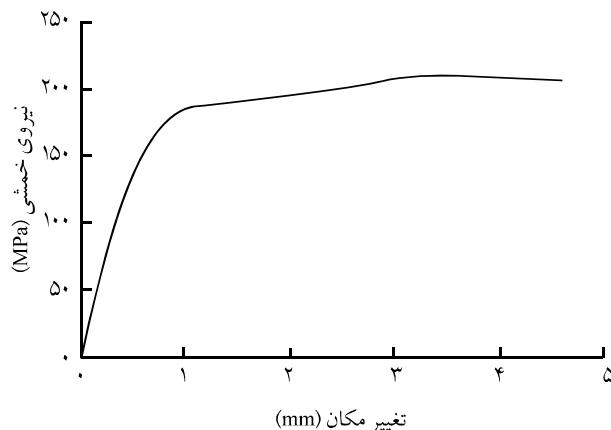
شکل ۱۰- رفتار مکانیکی نیروی خمشی در برابر انحنای نمونه ۳.
