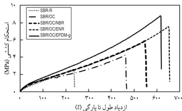
شکل ۱۰ - استحکام کششی و ازدیاد طول تا پارگی برای آمیخته SBR فاقد هر نوع پرکننده و نمونه‌های نانوکامپوزیت SBR/OC سازگار شده و سازگار نشده.
