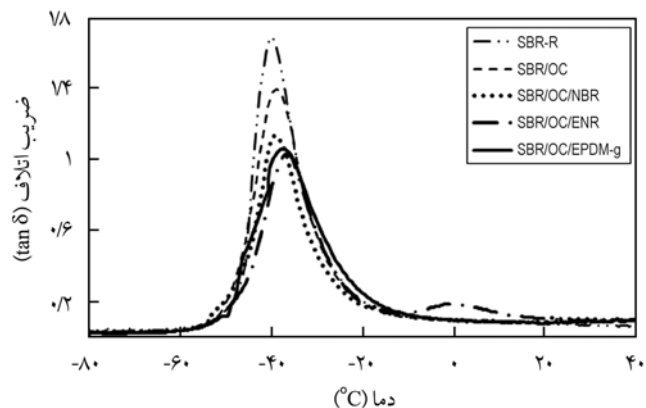
شکل ۹- ضریب اتلاف (tan δ) به عنوان تابعی از دما (T) برای آمیخته SBR فاقد هر نوع پرکننده و نمونه‌های نانوکامپوزیت SBR/OC سازگار شده و سازگار نشده.
