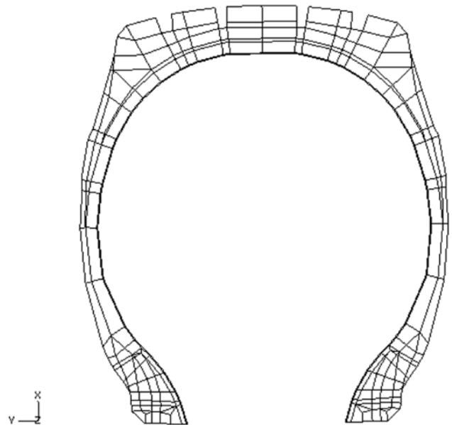
شکل ۲ - شبکه اجزای محدود دوبعدی تایلر.
