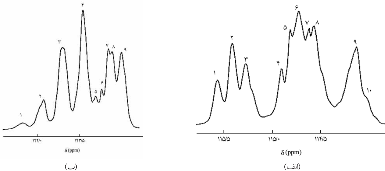
شکل ۵- طیف گسترده 13 C NMR نواحی کربن های اولفینی: (الف) متیلن و (ب) متین از ۲،۱- پلی بوتادی ان محلول در کلروفرم دوتریم دار در دمای ۲۰°C.
