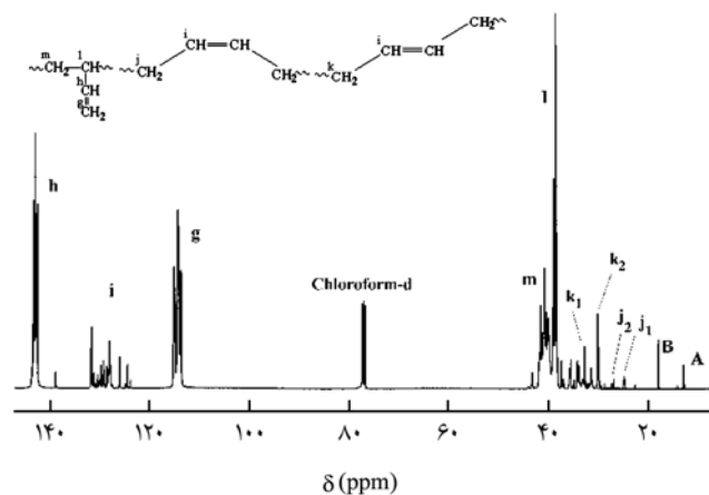
شکل ۲- طیف ^{13}\text{C} NMR از ۲،۱- پلی بوتادی ان در حلال کلروفرم دوتریم دار و در دمای 20^\circ\text{C} .
