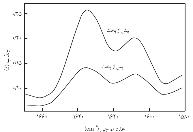
شکل ۱ - نمودار FTIR برای نمونه حاوی ۵ نانوذرات بوهمیت پیش و
