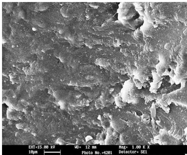
شکل ۷- تصویر SEM مربوط به سطح شکست نمونه حاوی ۰/۲ درصد وزنی پرکننده در آزمون استحکام خمشی.
