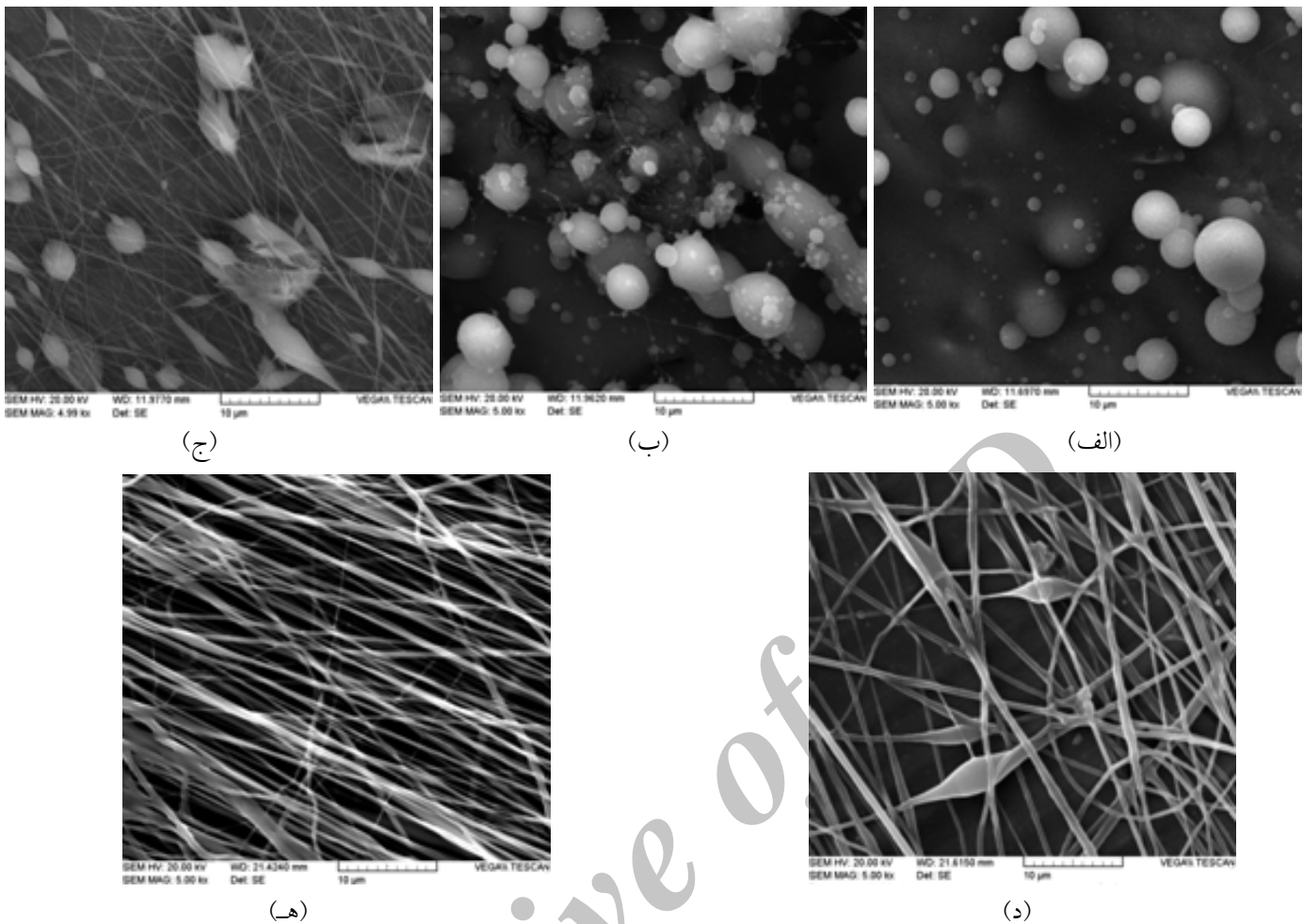
شکل ۳- تصاویر میکروسکوپ الکترونی پوشی PLGA الکتروریسی شده با سامانه‌های مختلف حلال و بزرگ‌نمایی ۵۰۰۰ برابر: (الف) DMF، (ب) DMF/THF، (ج) DMF- کلروفرم، (د) کلروفرم - متانول و (ه) HFIP.
