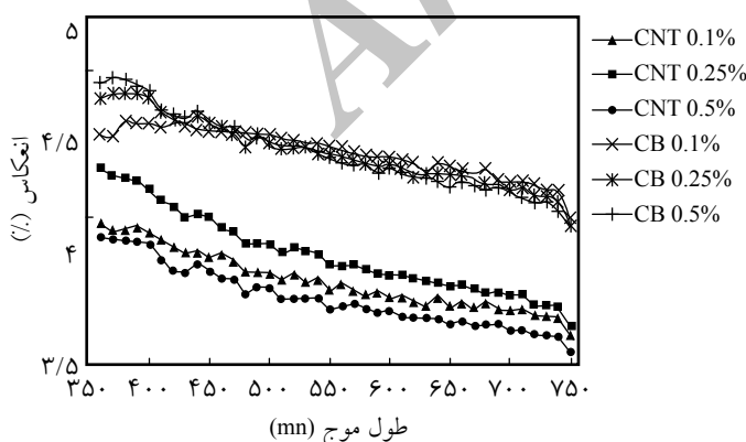
شکل ۲- طیف انعکاسی نانوکامپوزیت‌های پلی‌متیل متاکریلات حاوی ترکیب درصد‌های مختلفی از نانولوله‌های کربنی و کامپوزیت‌های حاوی دوده در ناحیه مرئی.
