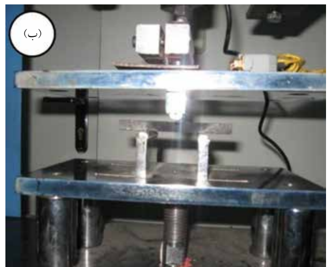
شکل ۶- نمایی از بست آزمون کشش و خمش استفاده شده.
