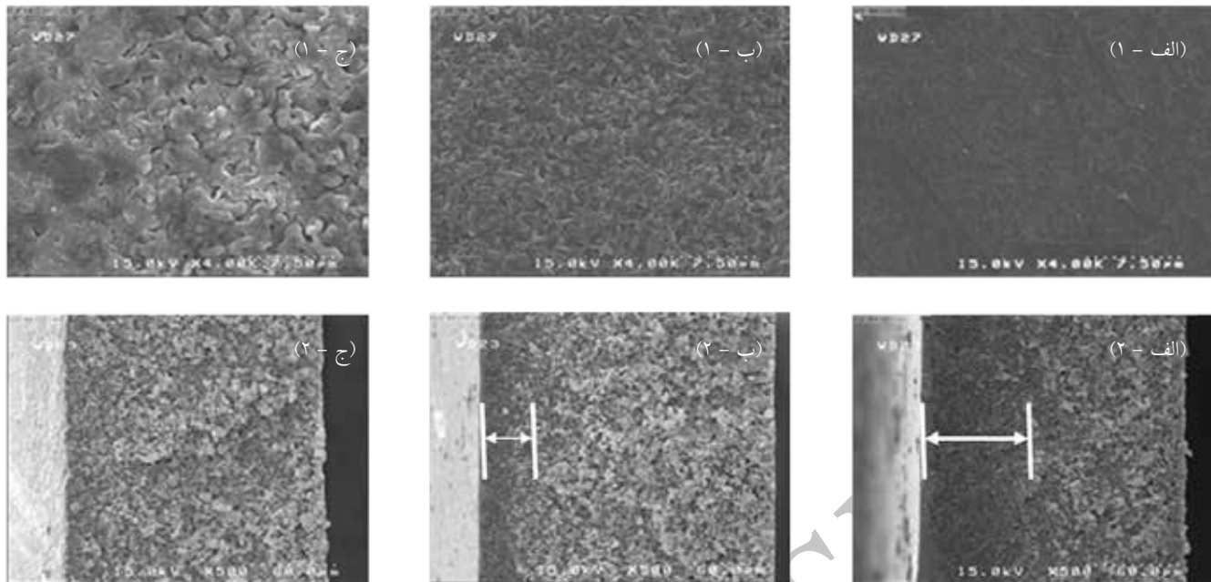
شکل ۲- تصاویر SEM غشای تخت ساخته شده با ۲۵٪ وزنی پلیمر در دماهای مختلف حمام انعقاد: (الف) ۰°C، (ب) ۳۰°C و (ج) ۶۰°C، (۱) سطح بیرونی غشا و (۲) سطح مقطع غشا.
