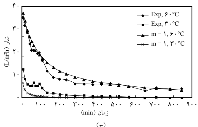
شکل ۶- بررسی سازوکار گرفتگی در غشاهای با تخلخل سطحی متفاوت و تطبیق داده‌های تجربی با سازوکار: (الف) m=2 گرفتگی کامل حفره، (ب) m=1/5 گرفتگی استاندارد حفره، (ج) m=1 گرفتگی متوسط حفره و (د) m=0 تشکیل لایه کیک.
