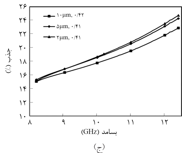
شکل ۸- تغییرات: (الف) بازتاب، (ب) عبور و (ج) جذب بر حسب بسامد نانوکامپوزیت اسفنجها در کسر حجمی ثابت (۰/۴۲ و ۰/۴۱) و اندازه سلولهای مختلف (حدود ۲، ۵ و ۱۰ μm).
