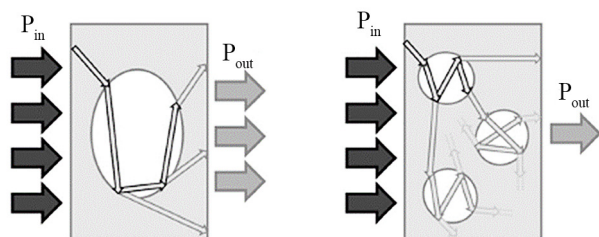
شکل ۱۰- تصویر کلی از پراکندگی های متعدد داخل اسفنج به سبب کاهش اندازه سلول.
