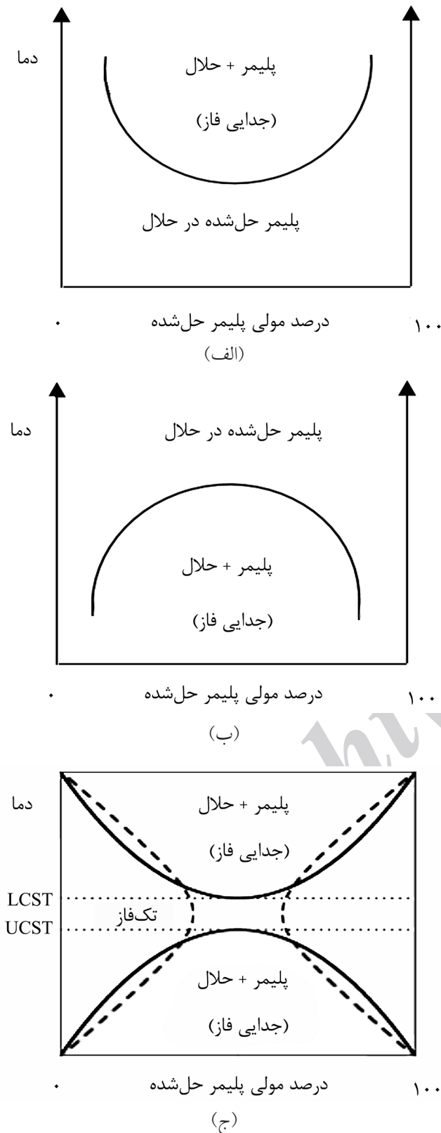
شکل ۱- نمودار تغییرات فاز پلیمرهای با رفتار گرمایی محلولی: (الف) LCST، (ب) UCST، (ج) UCST و LCST، (منحنی خطی باینودال و نقطه چین اسپینودال است) [۳۲].
