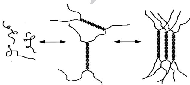
شکل ۳- تشکیل اتصالات فیزیکی در ژل در اثر تبدیل کلاف - ماریچ پس از کاهش دما [۲۸].
