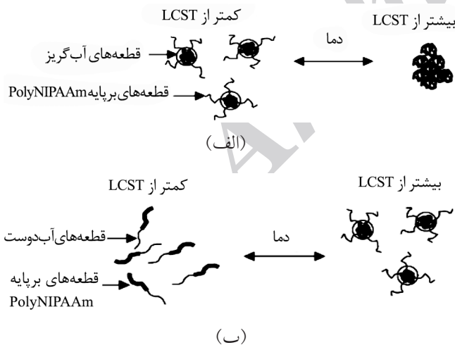
شکل ۱۱- دو نوع ساختار میسلی از کوپلیمر قطعه‌ای شامل یک بخش پلیمری پاسخگو به دما: (الف) کوپلیمر قطعه‌ای شامل پوسته بیرونی حساس به دما و هسته درونی آب‌گریز و (ب) کوپلیمر قطعه‌ای شامل هسته درونی حساس به دما و هاله بیرونی آب‌دوست [۱].
