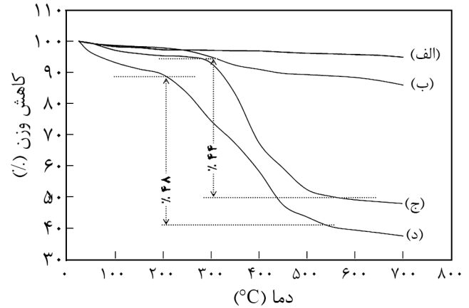
شکل ۲- دمانگاشت گرموزن‌سنجی: (الف) Fe_3O_4@SiO_2 ، (ب) Fe_3O_4@SiO_2 اصلاح‌شده با MPS، (ج) MNP@Pim و (د) MNP@PimSO_3H .
