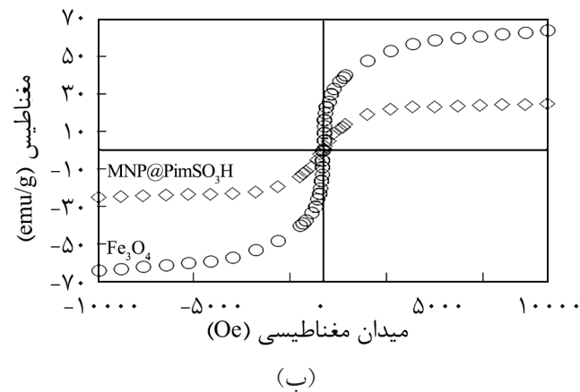
شکل ۳- (الف) الگوی XRD کاتالیزگر MNP@PimSO_3H و (ب) منحنی مغناطیس‌سنجی نانوذرات مغناطیسی خالص و کاتالیزگر MNP@PimSO_3H .
